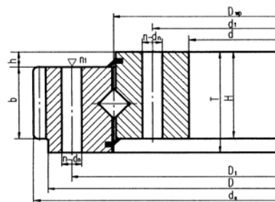
交叉圆柱滚子轴承外形尺寸
